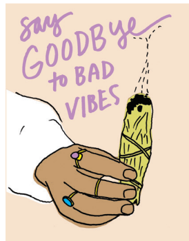
ct60 sage
